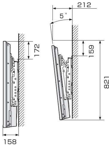
壁掛け金具AN-52AG6使用時
