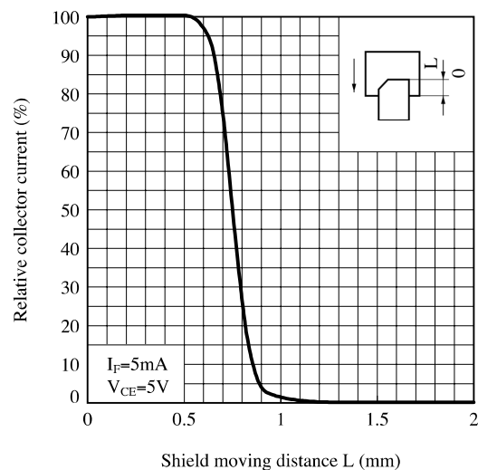
Fig.12 検出位置特性 (2)
