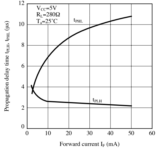
Fig.10 伝搬遅延時間—順電流特性
