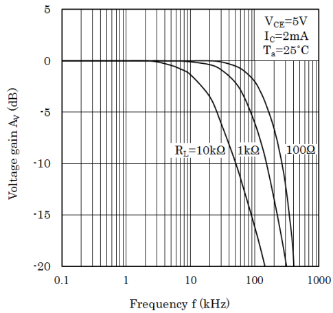
Fig.15 周波数特性
