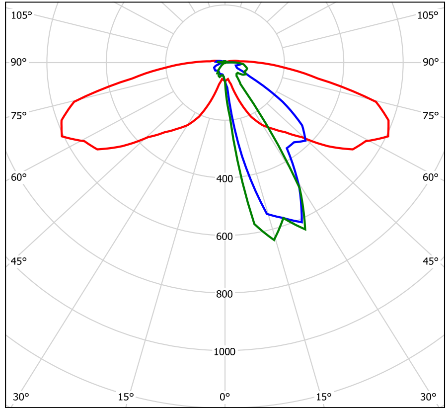
配光曲線(cd/1,000 lm)
