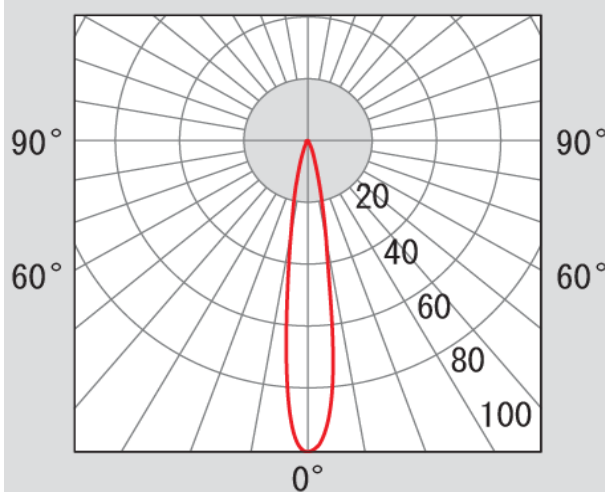
水平面照度 [lx] Ra84・14°
