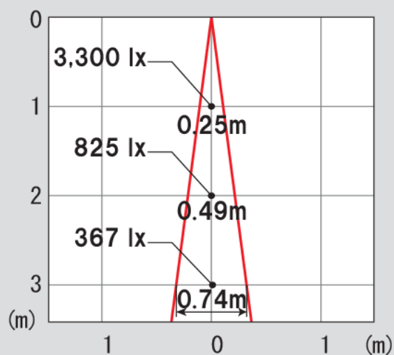
水平面照度 [lx] Ra84・14°
