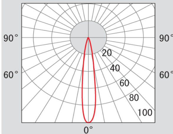
配光曲線 [%] Ra94・14°
