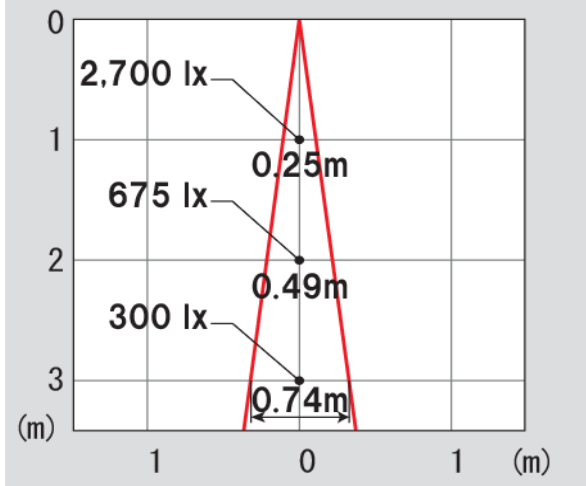
水平面照度 [lx] Ra94・14°
