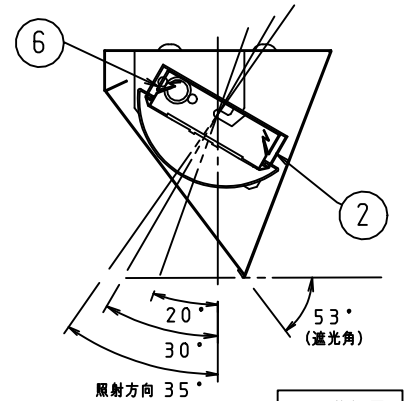
側面詳細図
