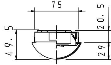
側面詳細図
