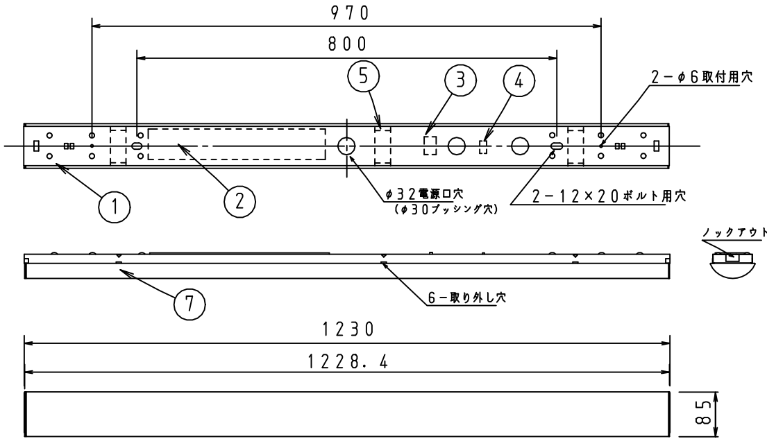
側面詳細図
