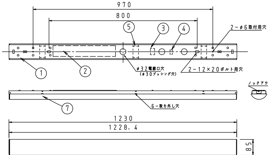
側面詳細図
