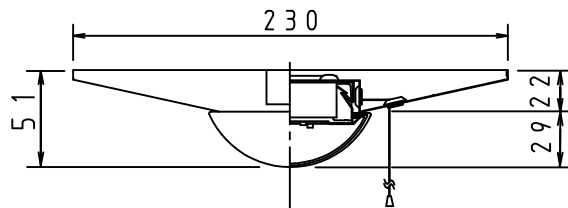
側面詳細図
