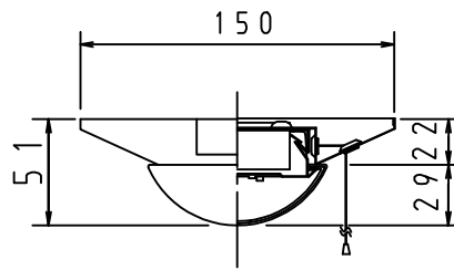
側面詳細図
