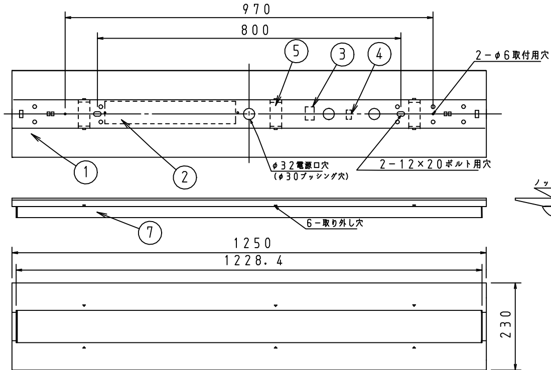
側面詳細図
