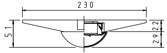
側面詳細図
