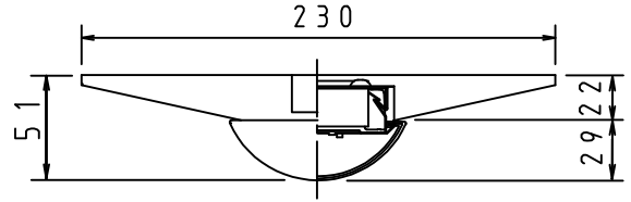
側面詳細図
