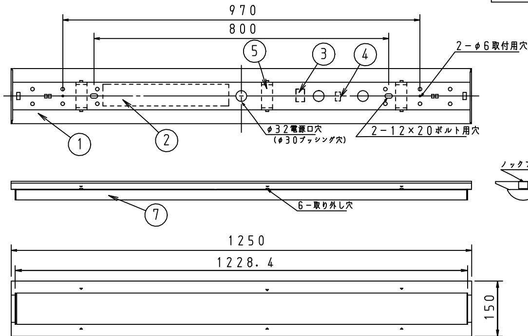
側面詳細図
