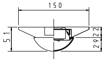
側面詳細図
