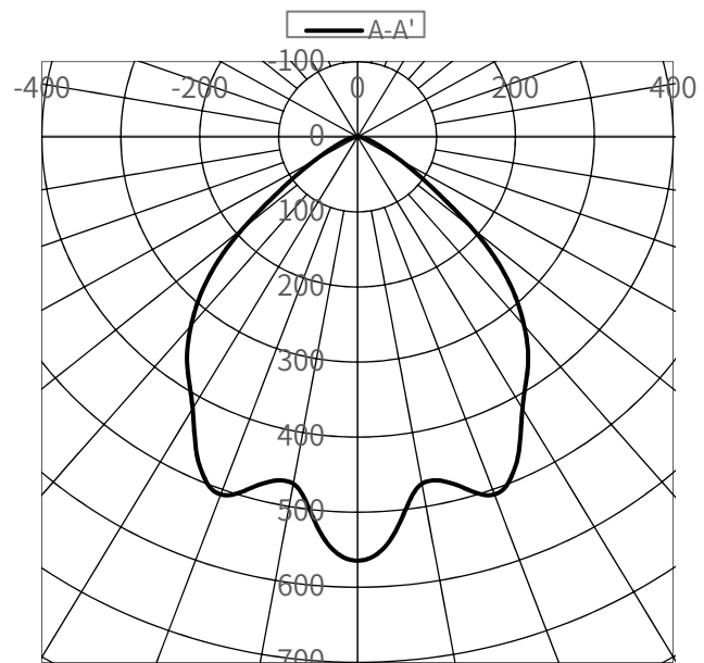
配光曲線(cd/1,000Lm)
