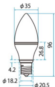
■ DL-JC2DL 寸法図
