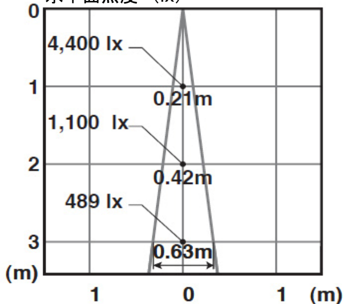
水平面照度 (lx)
