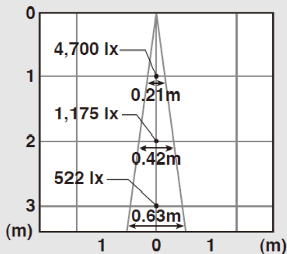
水平面照度[lx] Ra85・12°
