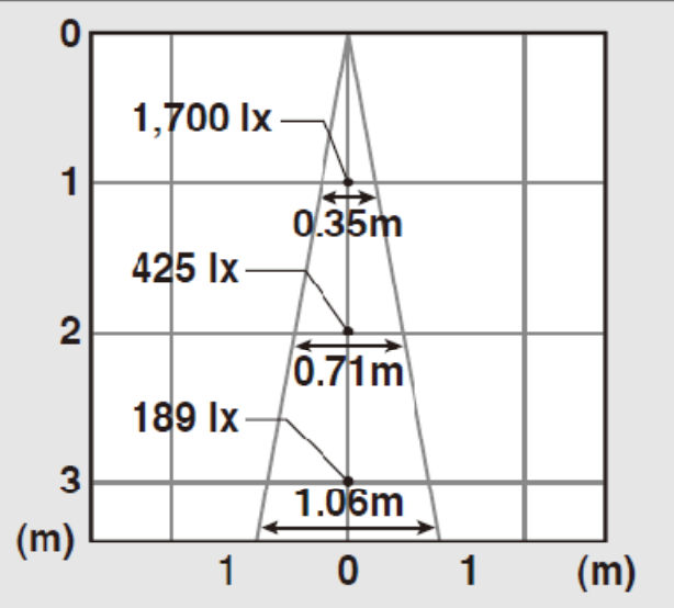
水平面照度[lx] Ra95・20°
