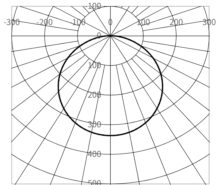
配光曲線(cd/1,000Lm)
