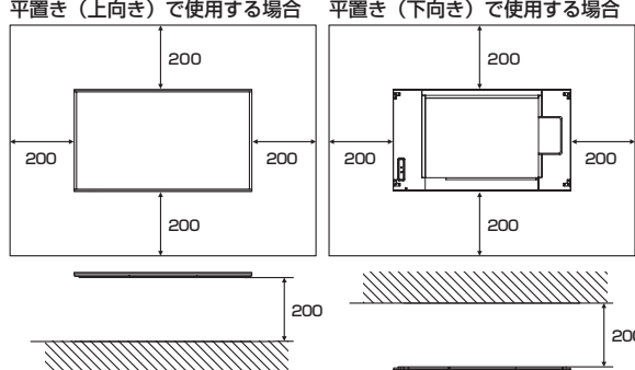
平置き（上向き）で使用する場合 平置き（下向き）で使用する場合 単位:mm
