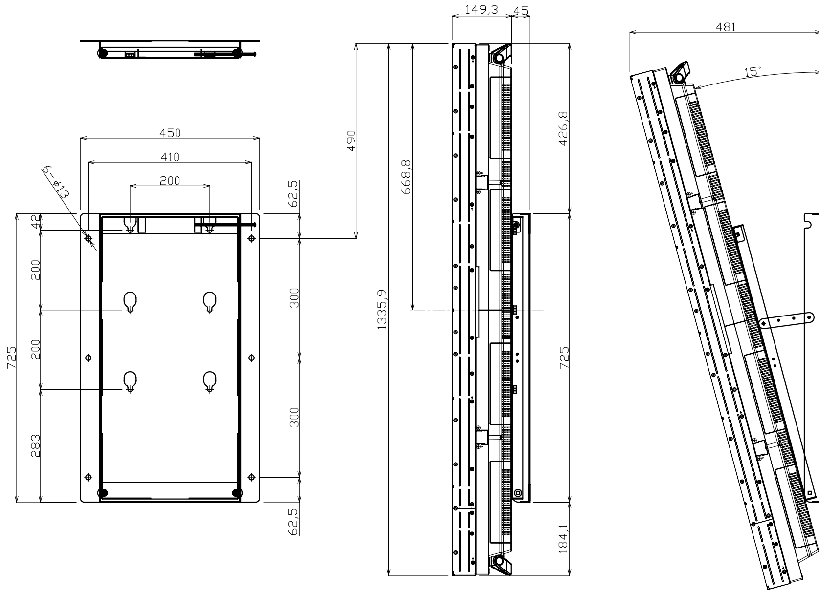
壁掛け金具 (PN-V602取付時) PN-ZK602 外観図
