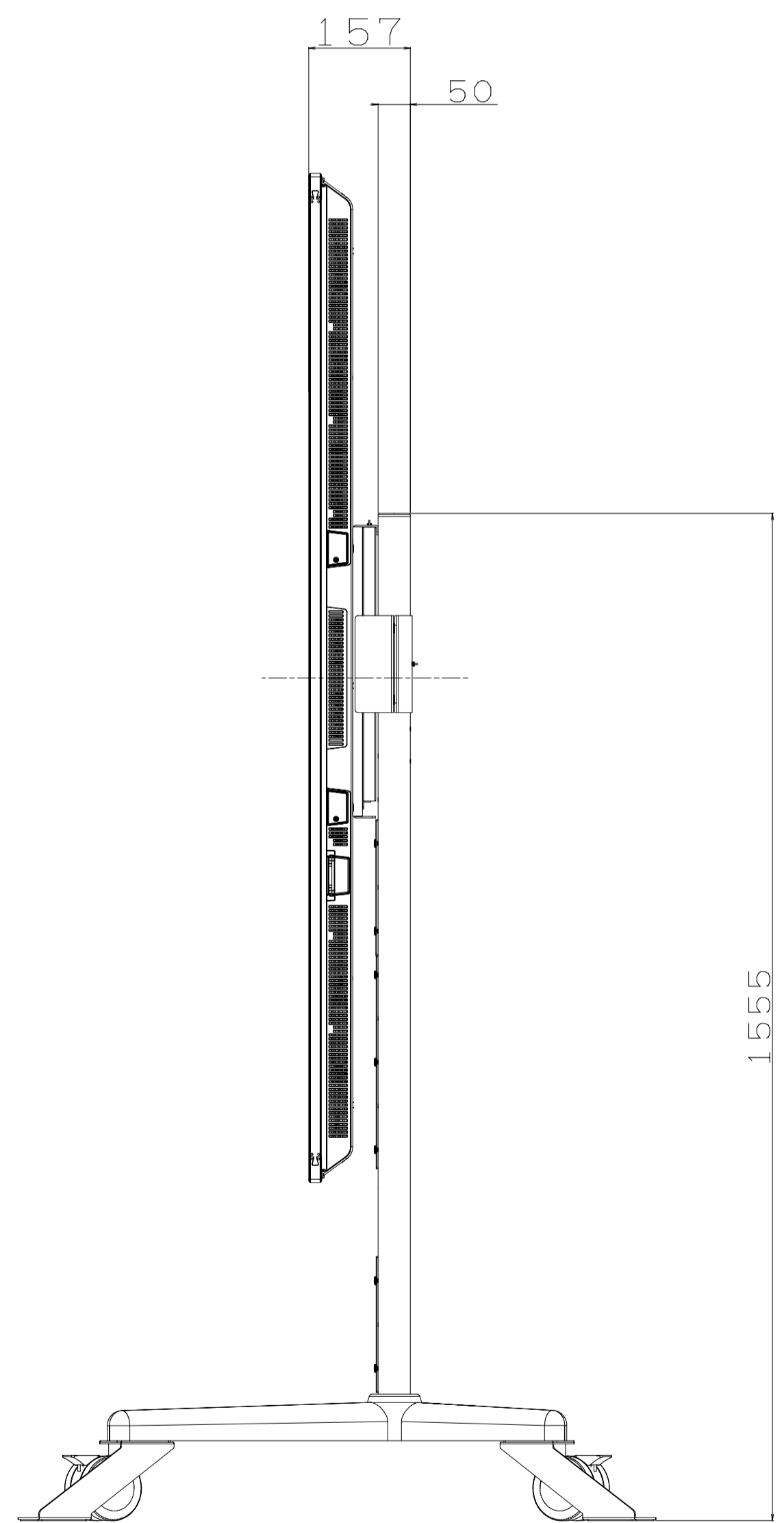
フロアスタンド (PN-H701 縦取付時) PN-ZS601 外観図
