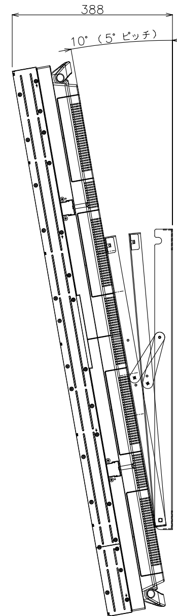
壁掛け金具 (PN-V601A取付時) PN-ZK602 外観図
