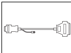
ZM-500CC (D-Sub9 ピン～ D-Sub25 ピン変換ケーブル) 0.3 m ZM-42 ～ 82 / ZM-300 シリーズの CN1 (D-Sub25 ピン) で使用していた通信ケーブルを、ZM-591XA の CN1 (D-Sub9 ピン) で使用するための変換ケーブルです。
